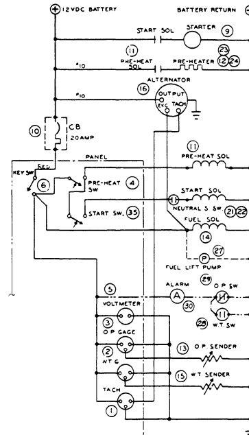
WATER TEMP. SWITCH (20) OIL PRESSURE SWITCH (20) ALARM (10) FUEL SOL. W58, W52, W70, W100 (14) FUEL LIFT PUMP (W51, W21, W27, W33, W52, W56, W70, W100 IF EQUIPPED) (27) PRE-HEATER (2) (24) OP SENDER (13) SEE NOTE-B (15) W T SENDER (16) ALTERNATOR (51 AMP) TACH (12) REG (11) PRE-HEAT SOL. (10) C B (20A) (9) STARTER (21) NEUTRAL SAFETY SWITCH (22) BATTERY RETURN (9) 12VDC (SEE NOTE-A) (2) (22) BATTERY (20) TACH (12) (14) (15) (16) (17) (18) (19) (20) (21) (22) (23) (24) (25) (26) (27) (28) (29) (30) (31) (32) (33) (34) (35) (36) (37) (38) (39) (40) (41) (42) (43) (44) (45) (46) (47) (48) (49) (50) (51) (52) (53) (54) (55) (56) (57) (58) (59) (60) (61) (62) (63) (64) (65) (66) (67) (68) (69) (70) (71) (72) (73) (74) (75) (76) (77) (78) (79) (80) (81) (82) (83) (84) (85) (86) (87) (88) (89) (90) (91) (92) (93) (94) (95) (96) (97) (98) (99) (100) NOT USED 15 SEE NOTE-B 16 ALTERNATOR 17 18 19 20 21 22 23 24 25 26 27 28 29 30 31 32 33 34 35 36 37 38 39 40 41 42 43 44 45 46 47 48 49 50 51 52 53 54 55 56 57 58 59 60 61 62 63 64 65 66 67 68 69 70 71 72 73 74 75 76 77 78 79 80 81 82 83 84 85 86 87 88 89 90 91 92 93 94 95 96 97 98 99 100 101 102 103 104 105 106 107 108 109 110 111 112 113 114 115 116 117 118 119 120 121 122 123 124 125 126 127 128 129 130 131 132 133 134 135 136 137 138 139 140 141 142 143 144 145 146 147 148 149 150 151 152 153 154 155 156 157 158 159 160 161 162 163 164 165 166 167 168 169 170 171 172 173 174 175 176 177 178 179 180 181 182 183 184 185 186 187 188 189 190 191 192 193 194 195 196 197 198 199 200 201 202 203 204 205 206 207 208 209 210 211 212 213 214 215 216 217 218 219 220 221 222 223 224 225 226 227 228 229 230 231 232 233 234 235 236 237 238 239 240 241 242 243 244 245 246 247 248 249 250 251 252 253 254 255 256 257 258 259 260 261 262 263 264 265 266 267 268 269 270 271 272 273 274 275 276 277 278 279 280 281 282 283 284 285 286 287 288 289 290 291 292 293 294 295 296 297 298 299 300 301 302 303 304 305 306 307 308 309 310 311 312 313 314 315 316 317 318 319 320 321 322 323 324 325 326 327 328 329 330 331 332 333 334 335 336 337 338 339 340 341 342 343 344 345 346 347 348 349 350 351 352 353 354 355 356 357 358 359 360 361 362 363 364 365 366 367 368 369 370 371 372 373 374 375 376 377 378 379 380 381 382 383 384 385 386 387 388 389 390 391 392 393 394
