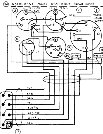
WATER TEMP. SWITCH (20) OIL PRESSURE SWITCH (20) ALARM (10) FUEL SOL. W58, W52, W70, W100 (14) FUEL LIFT PUMP (W51, W21, W27, W33, W52, W56, W70, W100 IF EQUIPPED) (27) PRE-HEATER (2) (24) OP SENDER (13) SEE NOTE-B (15) W T SENDER (16) ALTERNATOR (51 AMP) TACH (12) REG (11) PRE-HEAT SOL. (10) C B (20A) (9) STARTER (21) NEUTRAL SAFETY SWITCH (22) BATTERY RETURN (9) 12VDC (SEE NOTE-A) (2) (22) BATTERY (20) TACH (12) (14) (15) (16) (17) (18) (19) (20) (21) (22) (23) (24) (25) (26) (27) (28) (29) (30) (31) (32) (33) (34) (35) (36) (37) (38) (39) (40) (41) (42) (43) (44) (45) (46) (47) (48) (49) (50) (51) (52) (53) (54) (55) (56) (57) (58) (59) (60) (61) (62) (63) (64) (65) (66) (67) (68) (69) (70) (71) (72) (73) (74) (75) (76) (77) (78) (79) (80) (81) (82) (83) (84) (85) (86) (87) (88) (89) (90) (91) (92) (93) (94) (95) (96) (97) (98) (99) (100) NOT USED 15 SEE NOTE-B 16 ALTERNATOR 17 18 19 20 21 22 23 24 25 26 27 28 29 30 31 32 33 34 35 36 37 38 39 40 41 42 43 44 45 46 47 48 49 50 51 52 53 54 55 56 57 58 59 60 61 62 63 64 65 66 67 68 69 70 71 72 73 74 75 76 77 78 79 80 81 82 83 84 85 86 87 88 89 90 91 92 93 94 95 96 97 98 99 100 101 102 103 104 105 106 107 108 109 110 111 112 113 114 115 116 117 118 119 120 121 122 123 124 125 126 127 128 129 130 131 132 133 134 135 136 137 138 139 140 141 142 143 144 145 146 147 148 149 150 151 152 153 154 155 156 157 158 159 160 161 162 163 164 165 166 167 168 169 170 171 172 173 174 175 176 177 178 179 180 181 182 183 184 185 186 187 188 189 190 191 192 193 194 195 196 197 198 199 200 201 202 203 204 205 206 207 208 209 210 211 212 213 214 215 216 217 218 219 220 221 222 223 224 225 226 227 228 229 230 231 232 233 234 235 236 237 238 239 240 241 242 243 244 245 246 247 248 249 250 251 252 253 254 255 256 257 258 259 260 261 262 263 264 265 266 267 268 269 270 271 272 273 274 275 276 277 278 279 280 281 282 283 284 285 286 287 288 289 290 291 292 293 294 295 296 297 298 299 300 301 302 303 304 305 306 307 308 309 310 311 312 313 314 315 316 317 318 319 320 321 322 323 324 325 326 327 328 329 330 331 332 333 334 335 336 337 338 339 340 341 342 343 344 345 346 347 348 349 350 351 352 353 354 355 356 357 358 359 360 361 362 363 364 365 366 367 368 369 370 371 372 373 374 375 376 377 378 379 380 381 382 383 384 385 386 387 388 389 390 391 392 393 394
