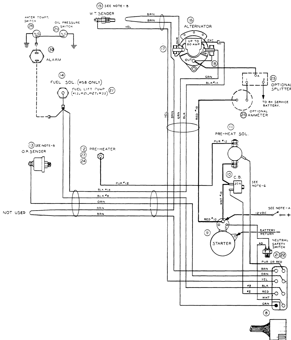
WIRING DIAGRAM.
