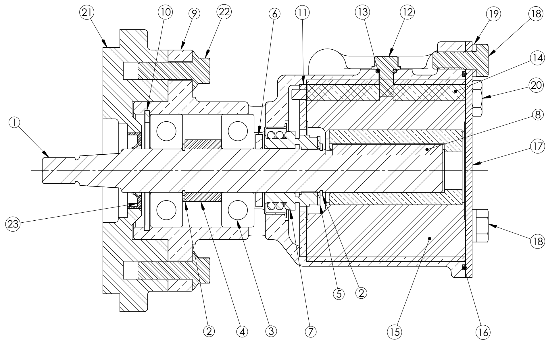
SECTION A-A
